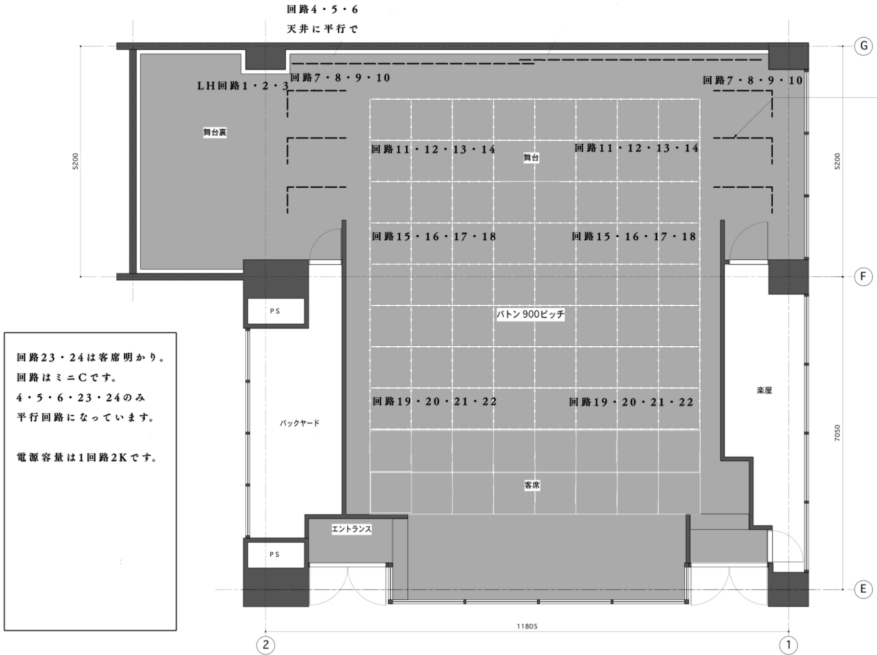
甘棠館照明図面
